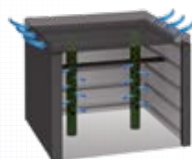
A központilag elhelyezett szellőzőcsövek biztosítják az optimális oxigénellátást és a légkeverést, mely által hatékony komposztálási folyamat jön létre.
