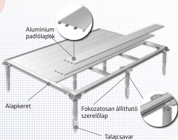
Kép: Talajcsavar - alap
