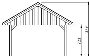
zijzicht 360
